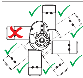
Von Lofrans entwickeltes Marine- Aluminium-Getriebe Installation positions
