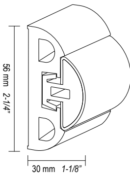
BINOX 35
