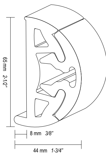
BINO 65
