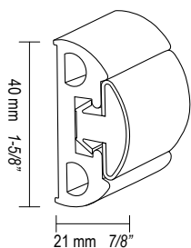
BINOX 25
