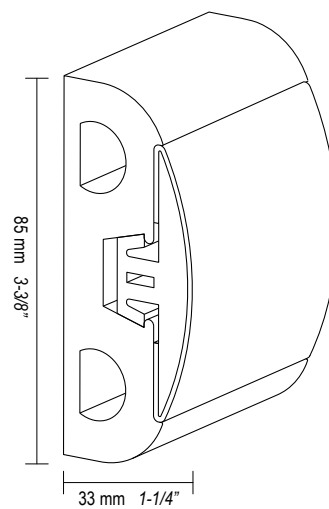
BINOX 65
