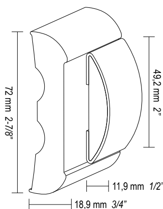
SPHÆRA 50
