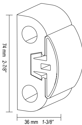
BINOX 50
