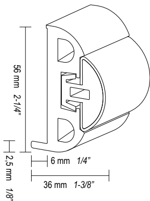
BINOX 35
