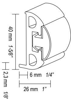
BINOX 25
